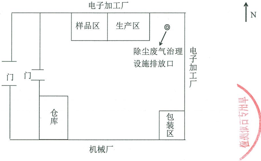
固定污染源有组织排放废气测点示意图
